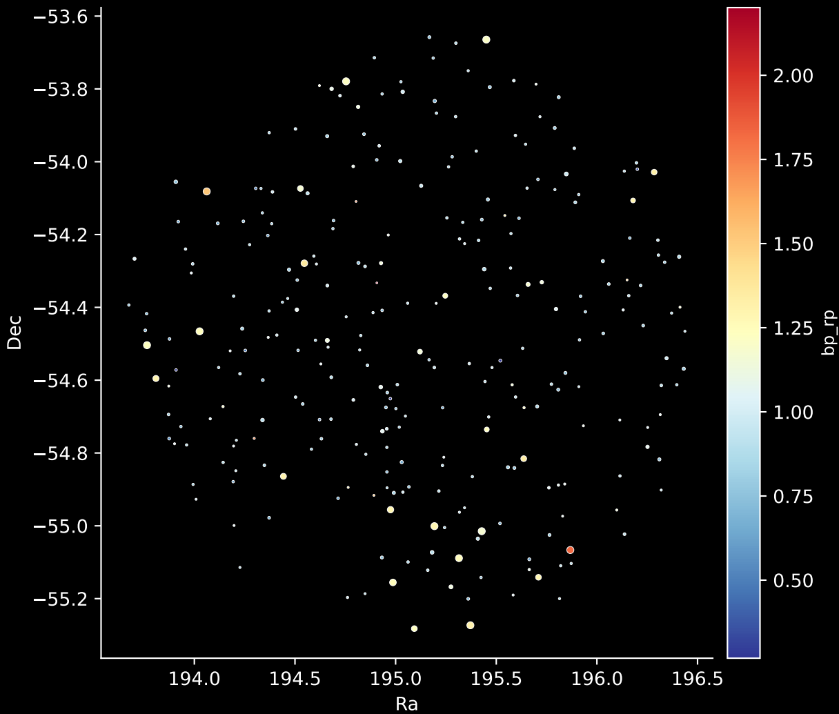
GALAH DR4 Field: [1277] Stars: 278
