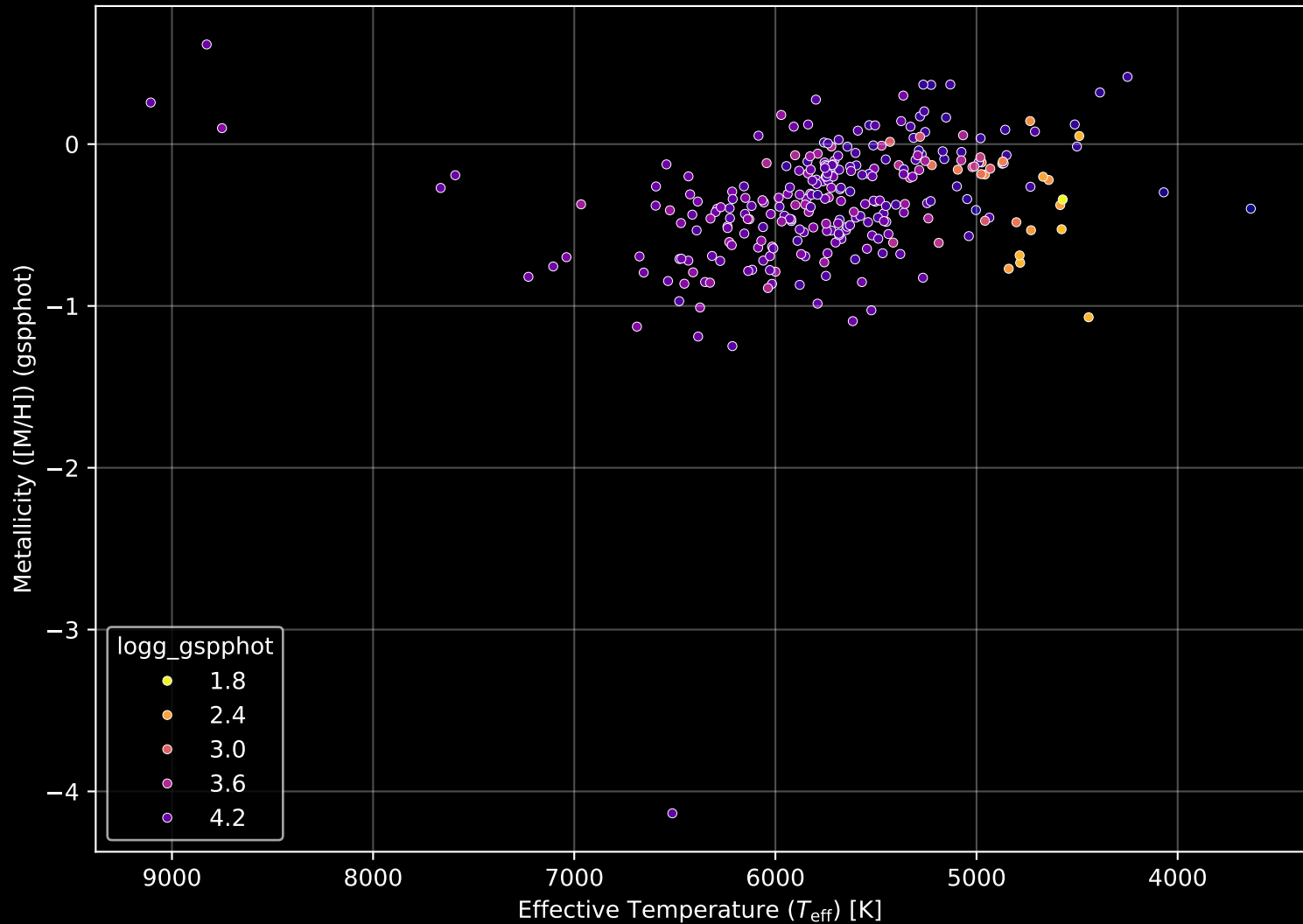
GALAH DR4 Field: [1277] Stellar Population Parameters (n= 278)
